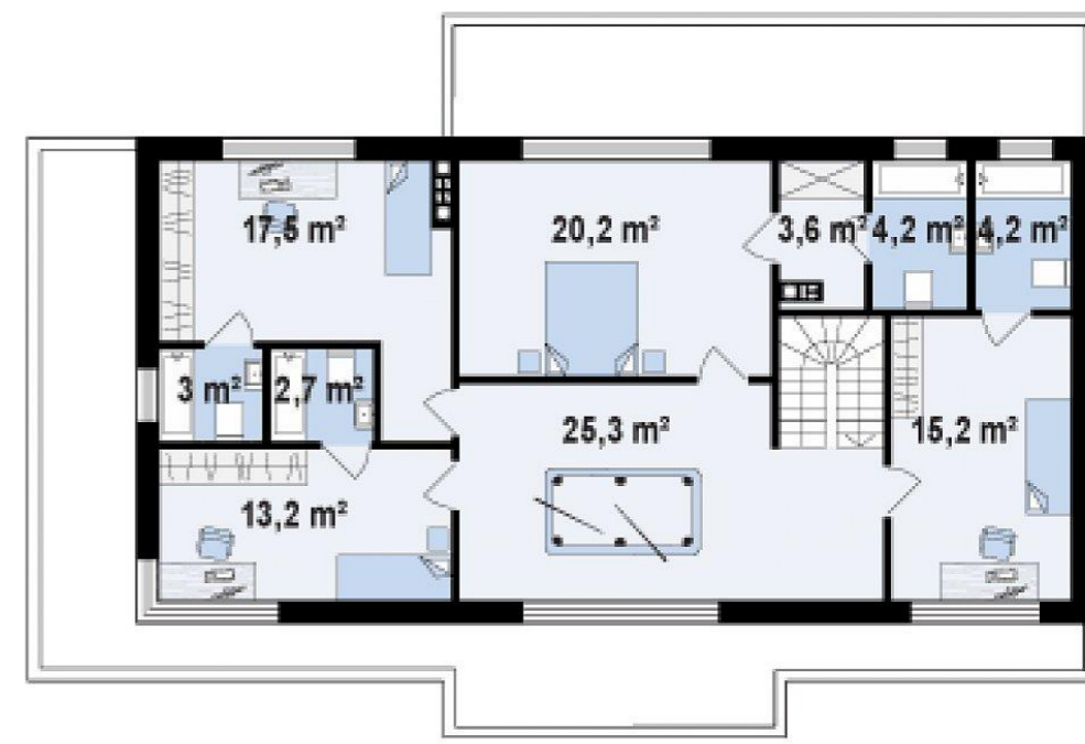
План 2 этаж
