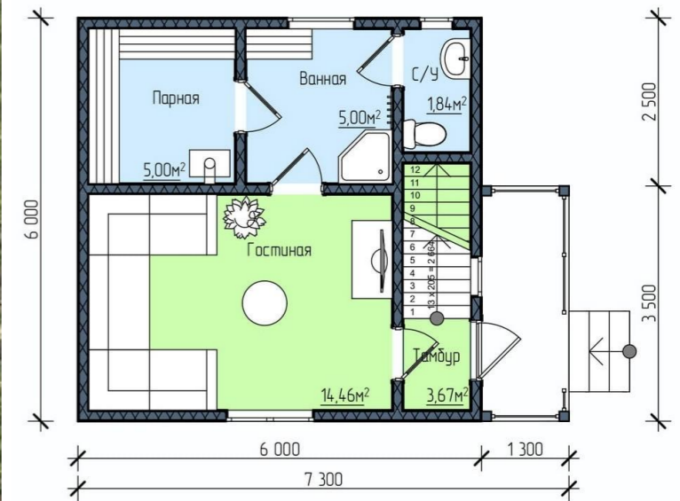
План 1 этаж
