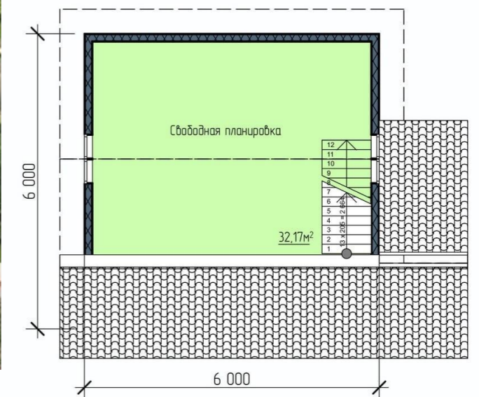
План 2 этаж
