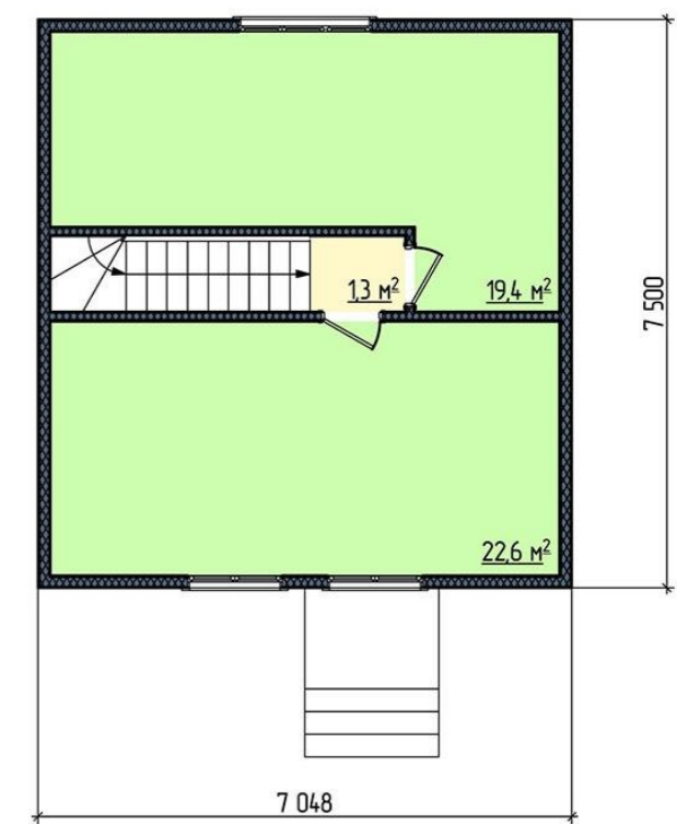
План 2 этаж
